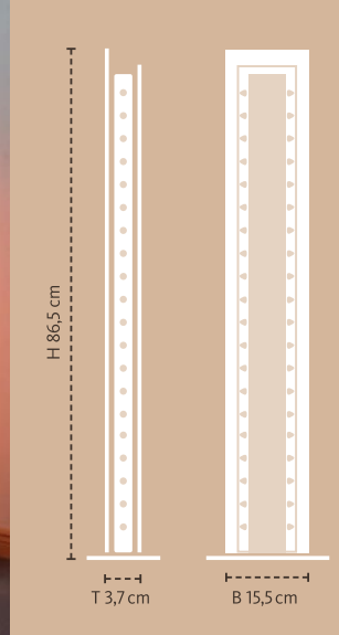
Seiten- und Frontansicht Akki 40 AF
