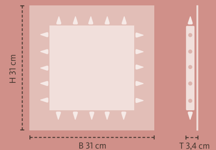
Front- und Seitenansicht Akki 20
